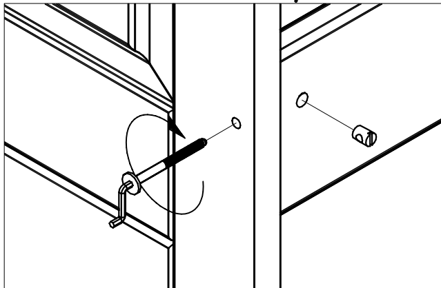
Монтаж царг
