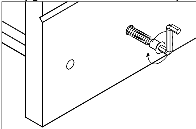
Закручивание стяжки-саморез
