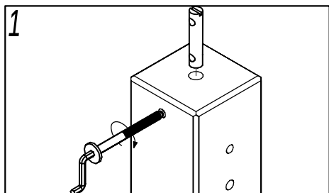
Крепление лестницы
