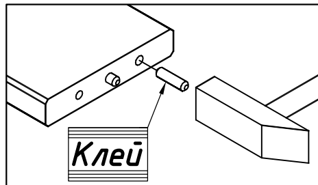
Забивание шкантов
