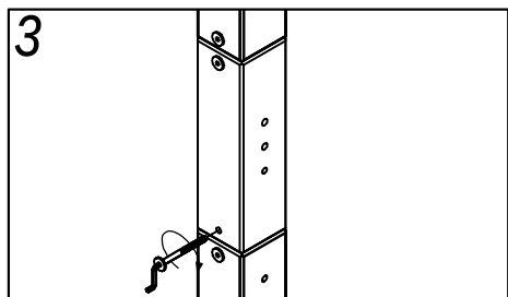
Крепление настила
