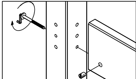
Крепление царг
