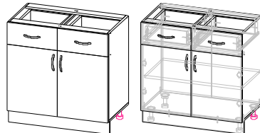
C2Я-800 (800x806x445мм)
