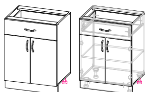
C1Я-600 (600x806x445мм)
