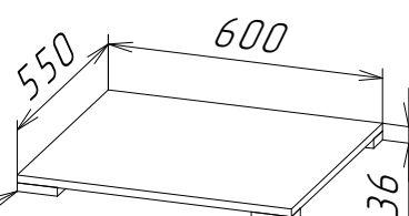
Модуль ГП-600
